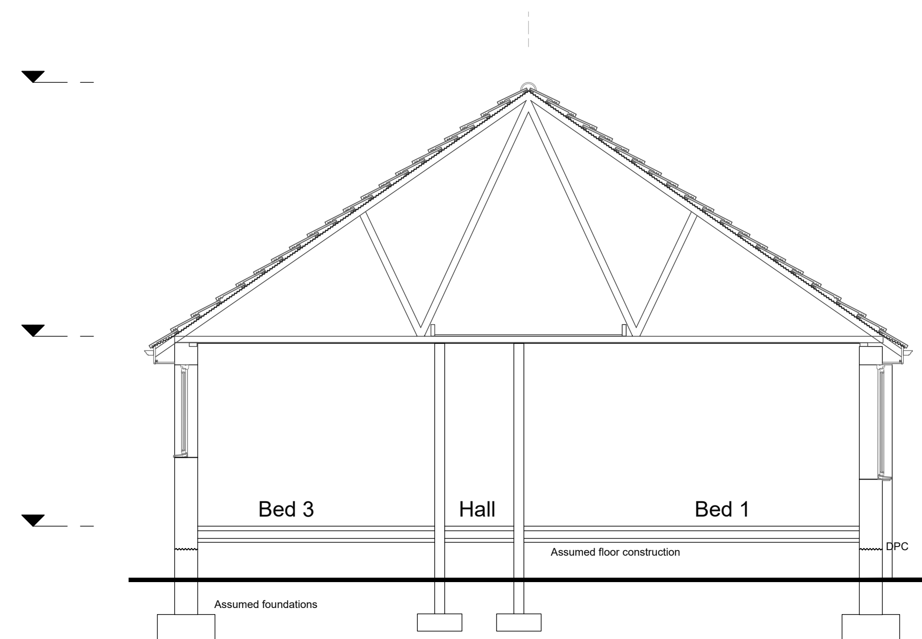
Section A-A 1:50
