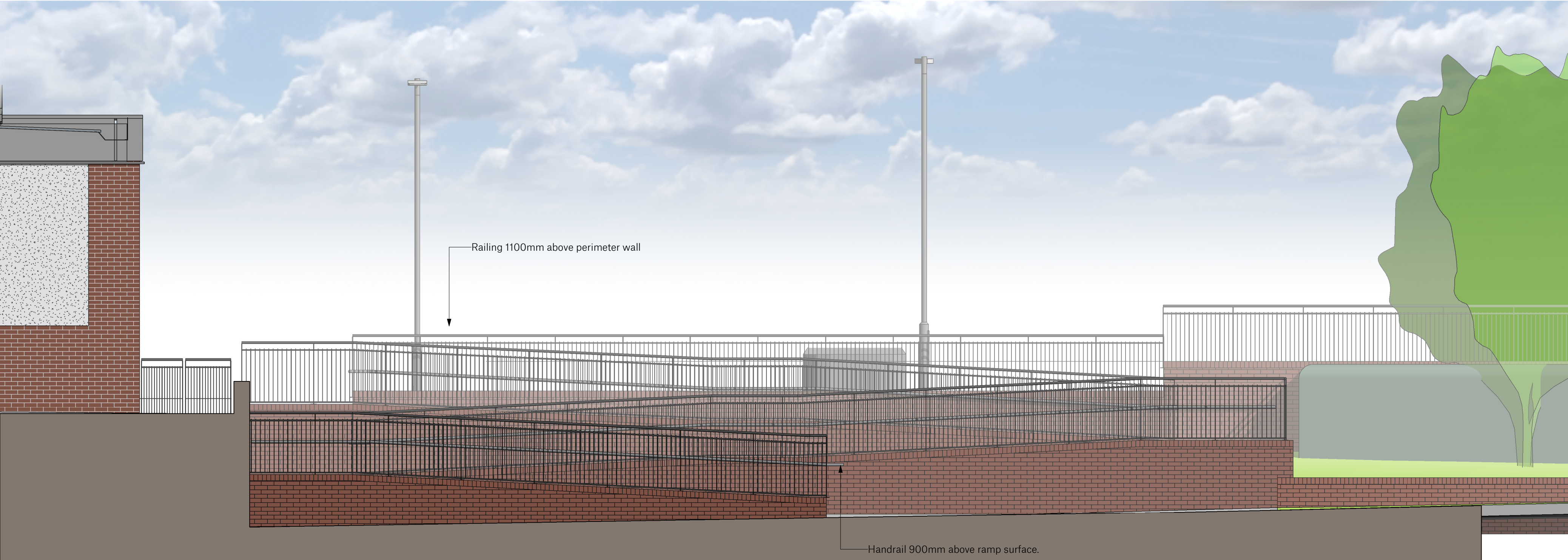
Ramp Elevation 1:50
